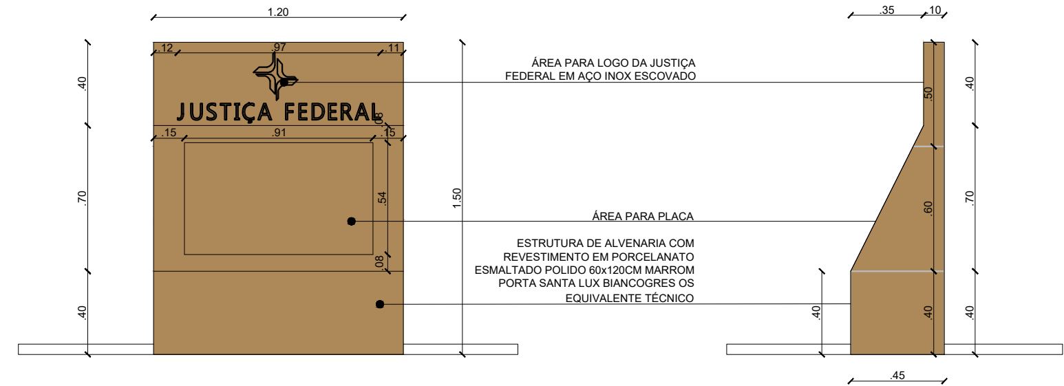
VISTA FRONTAL esc 1:25
