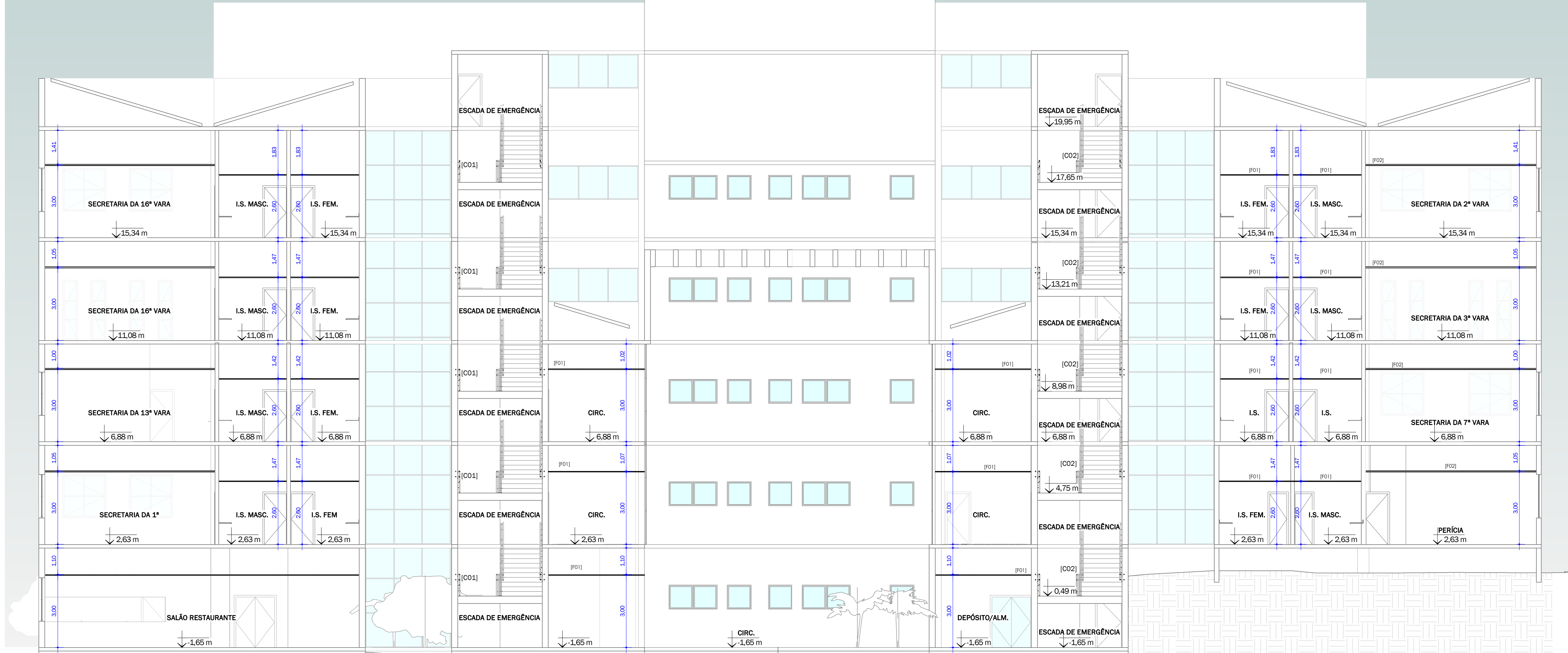
EDF. SEDE - CORTE AA' ESCALA 1:100
