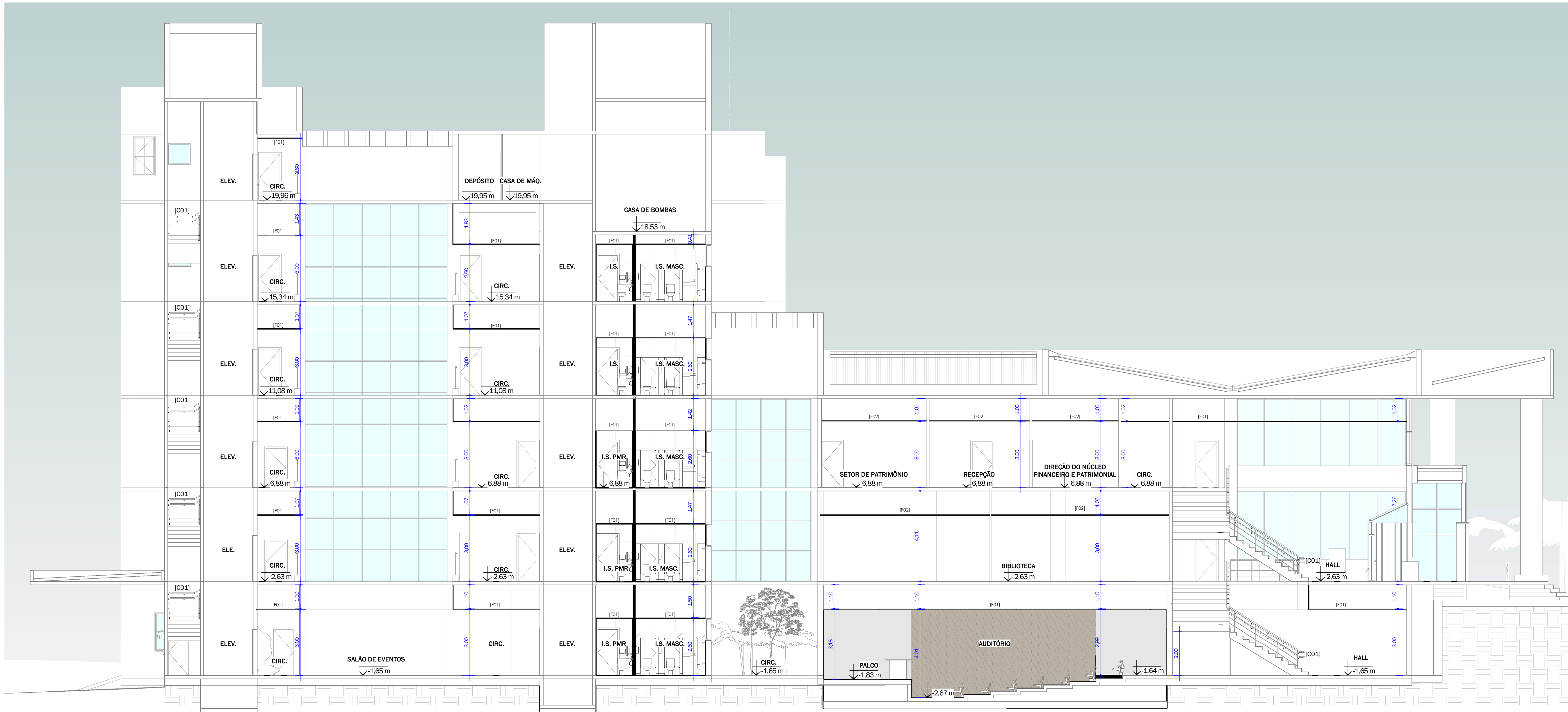
EDF. SEDE - CORTE BB' ESCALA 1:100
