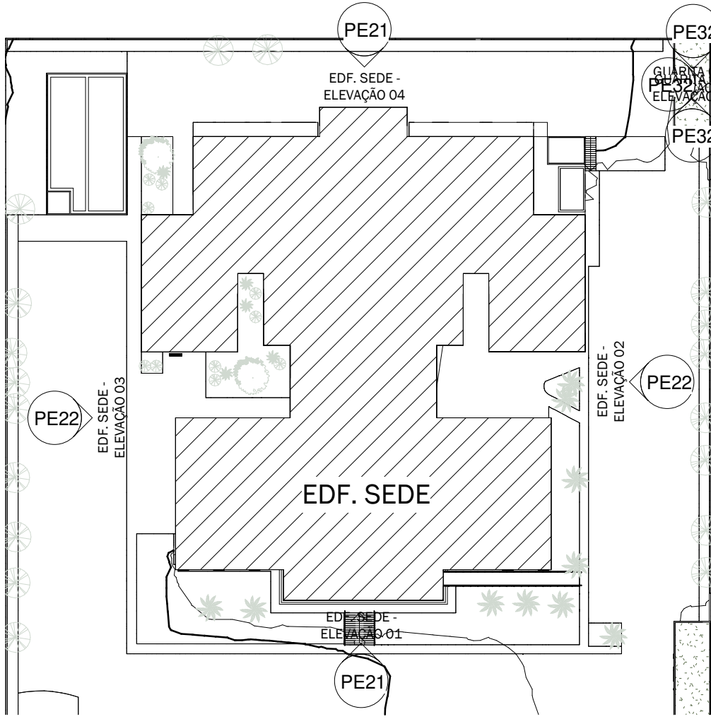
PLANTA CHAVE ESCALA 1:750
