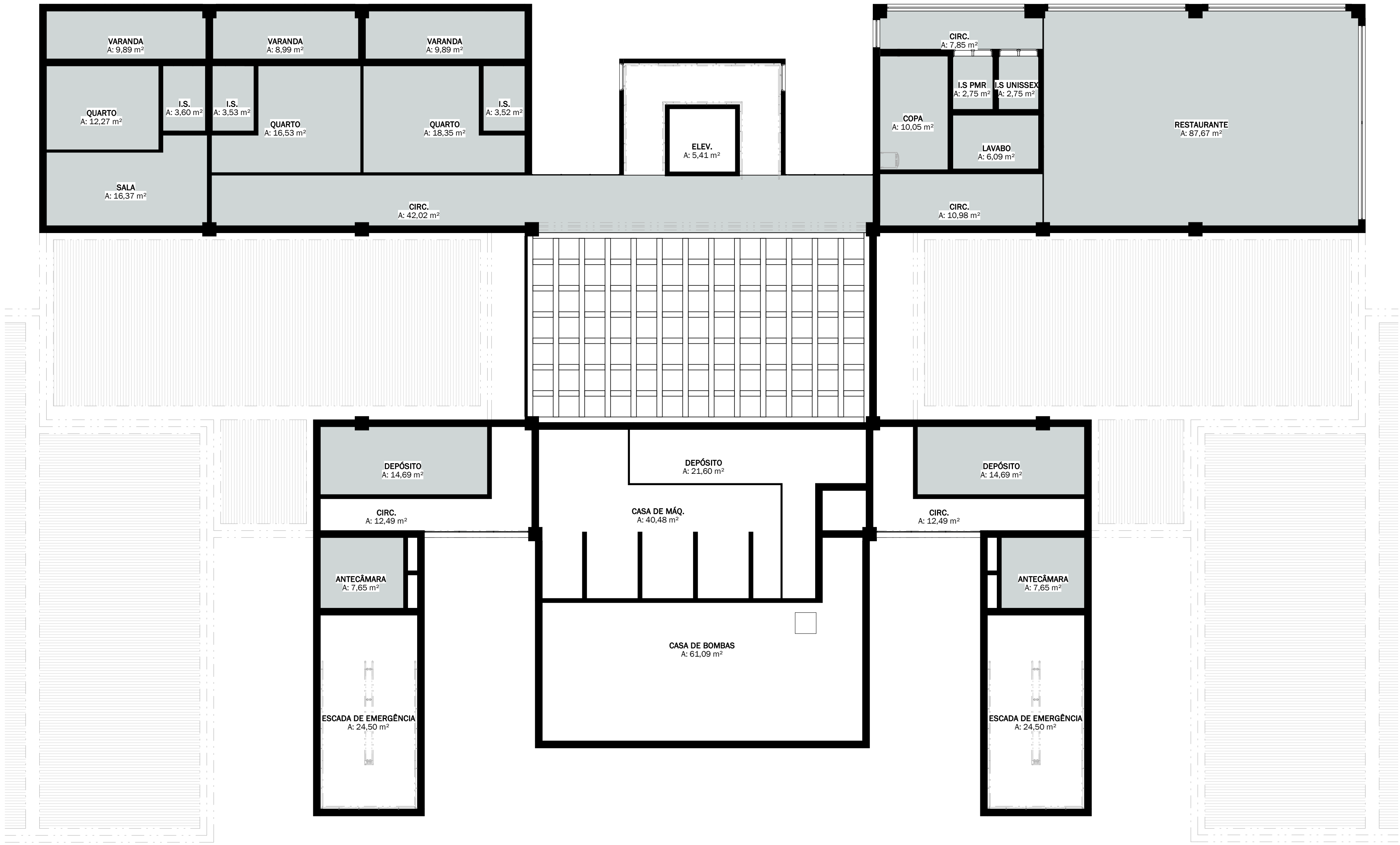
EDF. SEDE - PLANTA DE FORRO - PAV. 04 ESCALA 1 : 100
