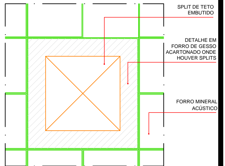
FORRO DE GESSO | DETALHE 03 1/25
