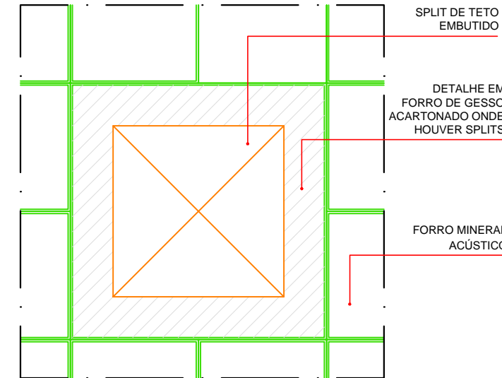
FORRO DE GESSO | DETALHE 03 1/25
