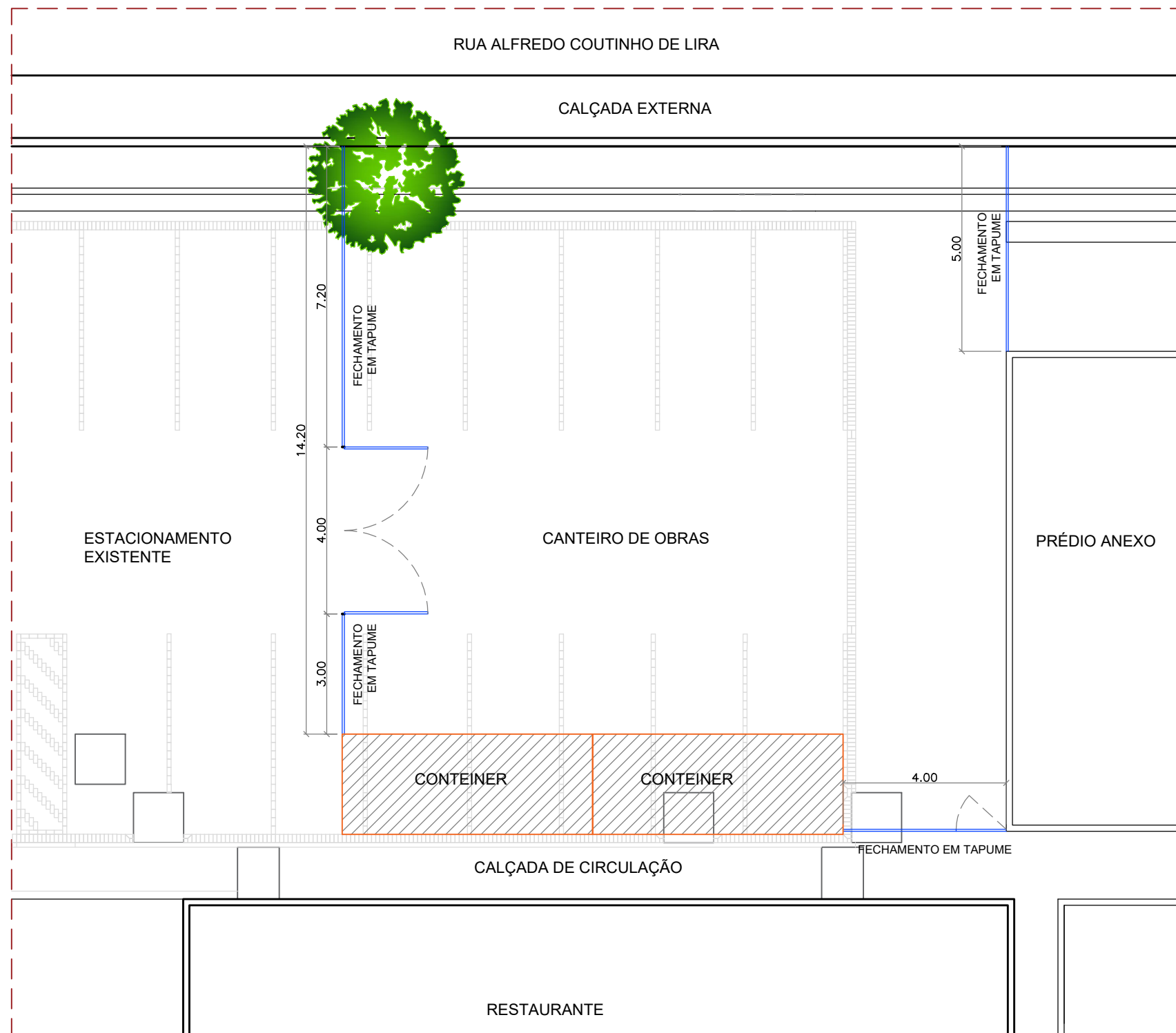
PLANTA BAIXA - CANTEIRO ESCALA 1:125
