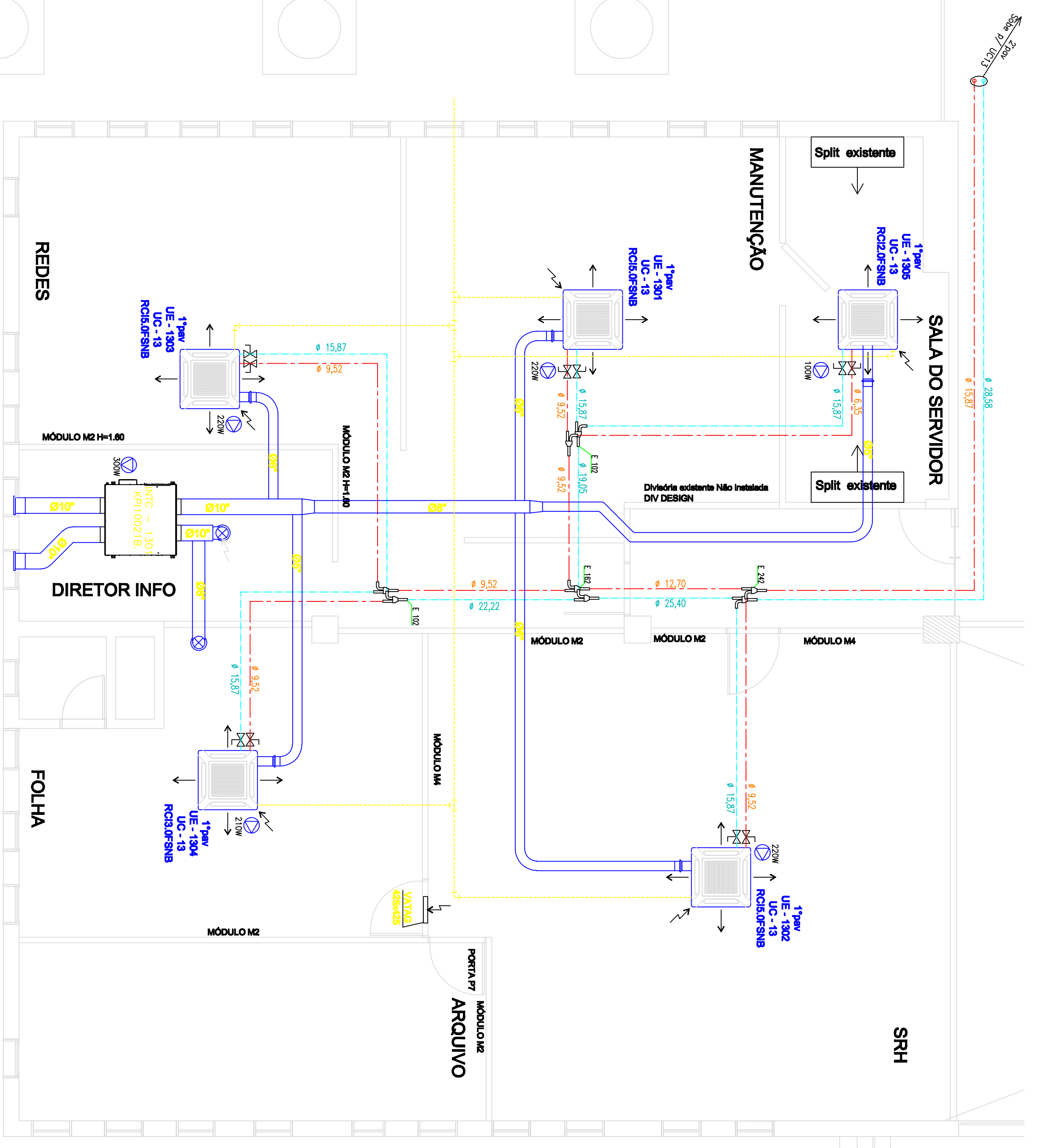
PLANTA BAIXA SET FREE - SGP/INFORMÁTICA ESCALA 1/50
