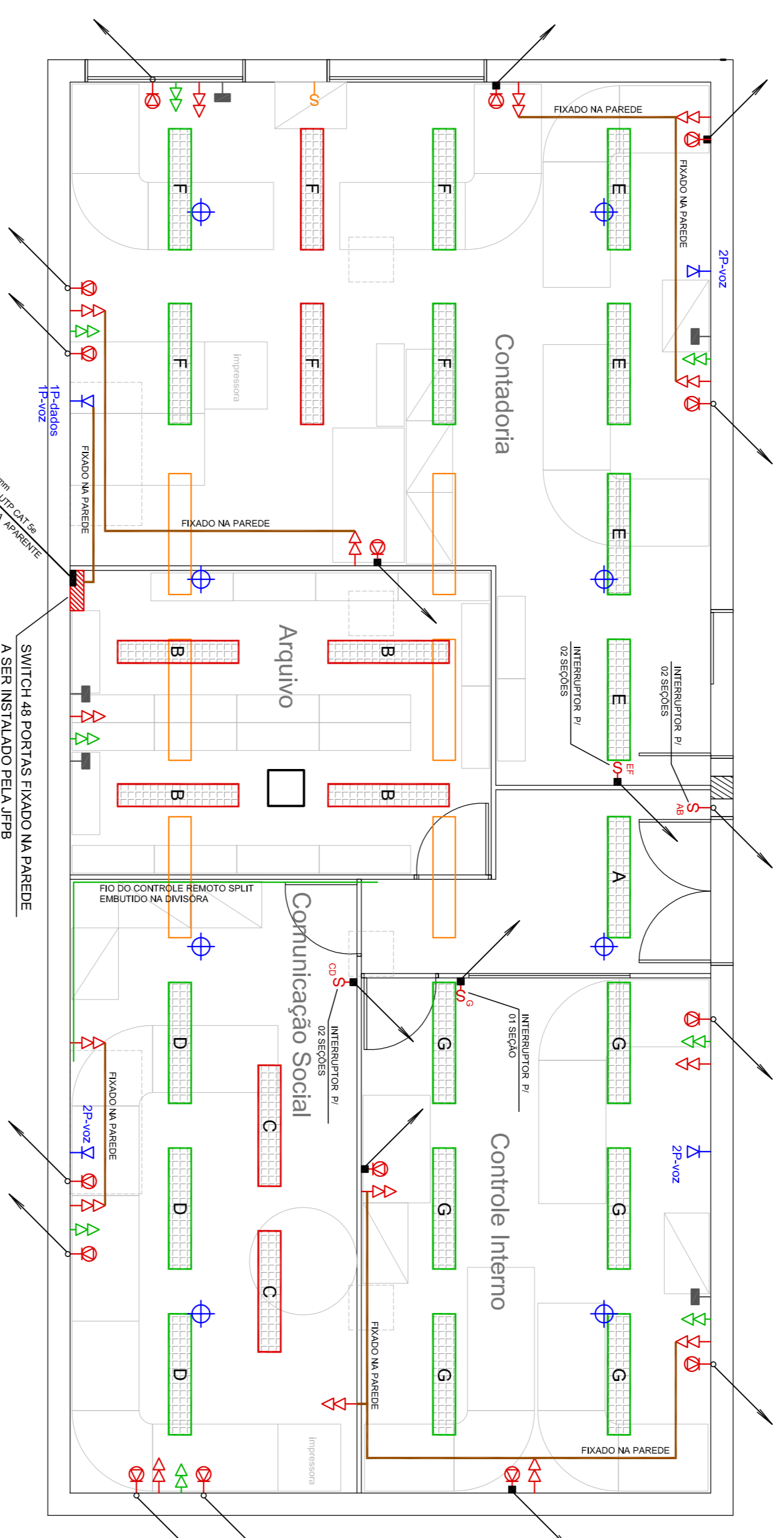
PLANTA BAIXA - PONTOS ELÉTRICOS/LÓGICOS ESCALA 1/50
