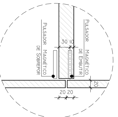
DETALHE 04 Armário 01 ESCALA 1/5
