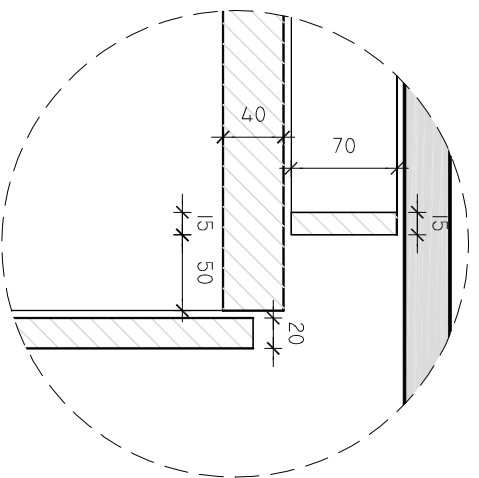
DETALHE 03 Armário 01 ESCALA 1/5
