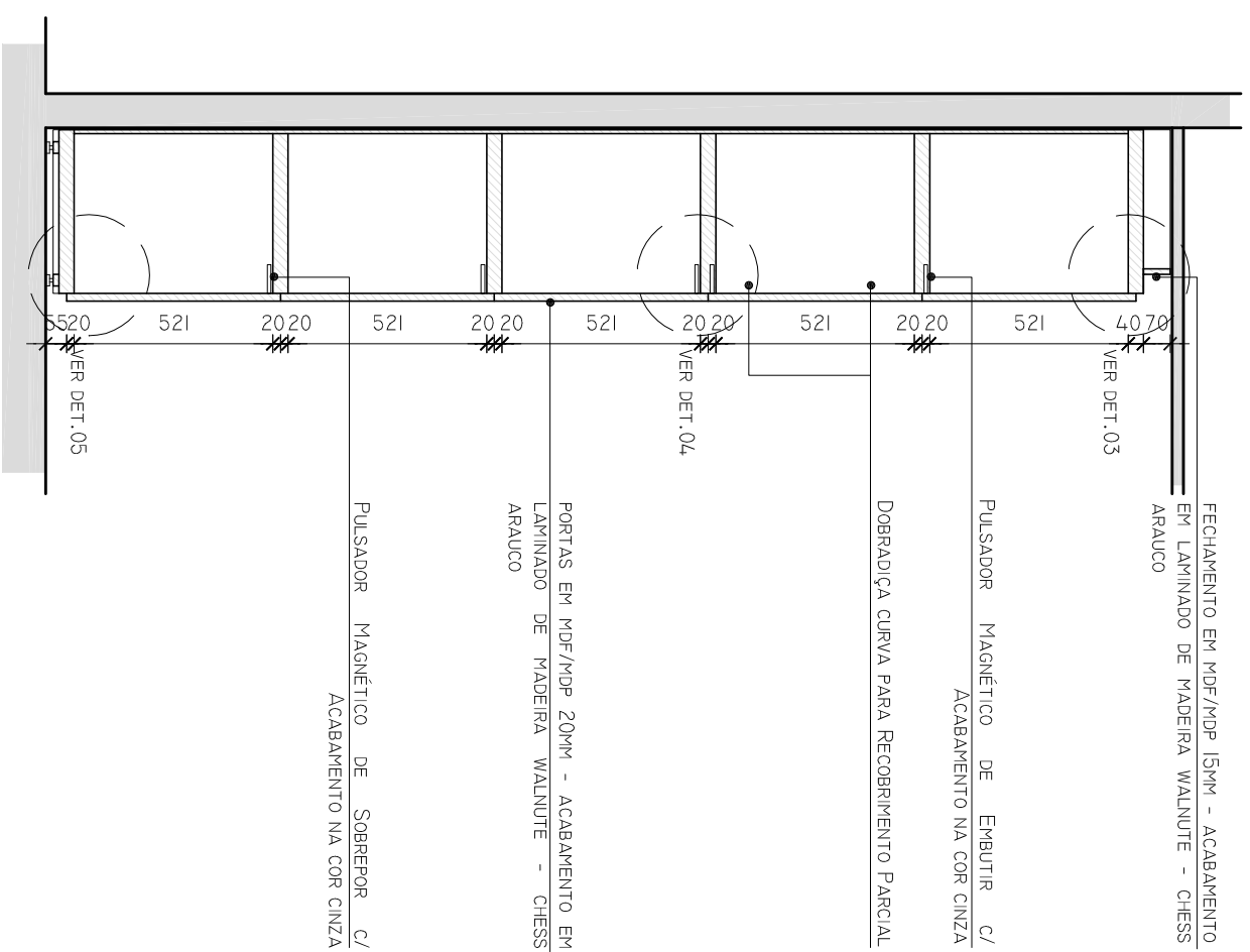
CORTE AA Armário 01 ESCALA 1/20
