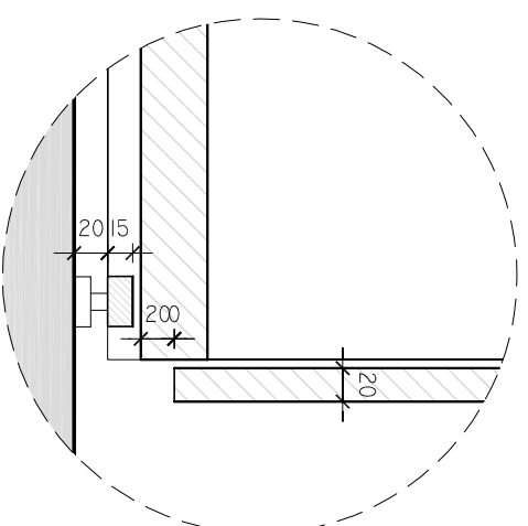
DETALHE 05 Armário 01 ESCALA 1/5
