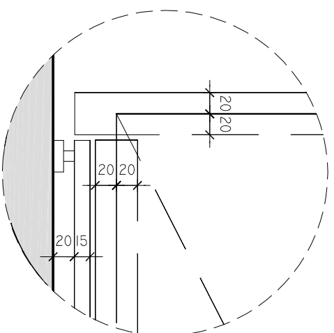
DETALHE 01 Armário 01 ESCALA 1/5
